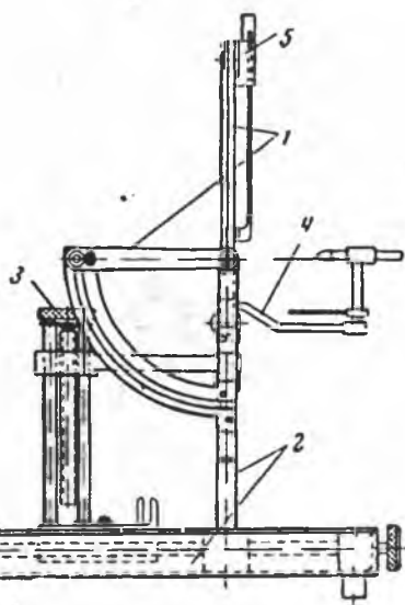
Рис. 26. Краниометр
