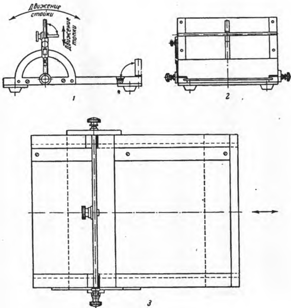
Рис. 7. Мандибулометр
