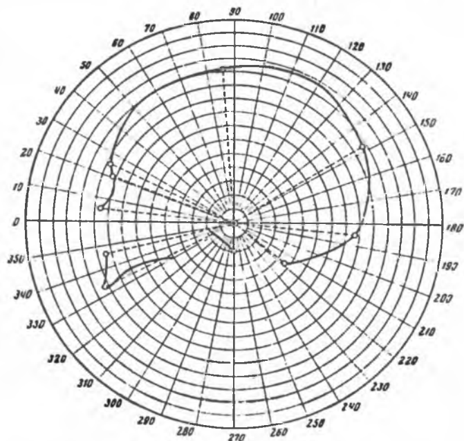
Рис. 34. «Круговой» график для вычисления среднего контура с интервалами 10^\circ и 10 мм
