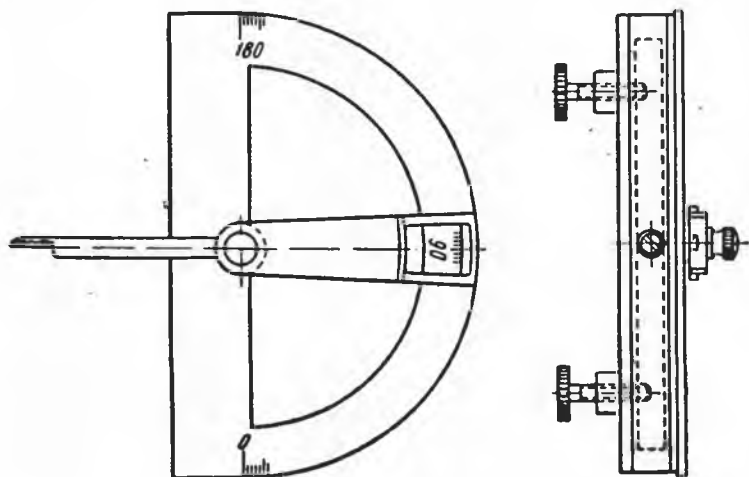
Рис. 6. Гониметр. Вид спереди и сбоку
