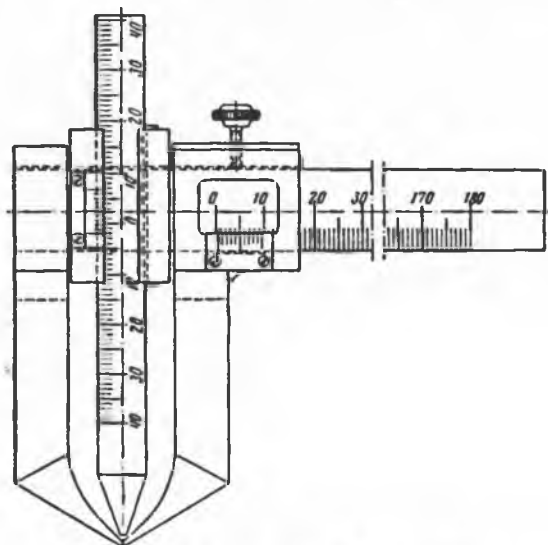
Рис. 3. Координатный циркуль
